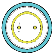
A: ECU电源 1: 电源正极 2: 电源负极
