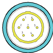
B: ECU数据连接 1: 三段开关 数据 2: 油门 三段开关 共正极6V 3: RX232 TX 4: RX232 GND 5: RX232 RX 6: 油门 数据 7: 油门 三段开关 共负极
